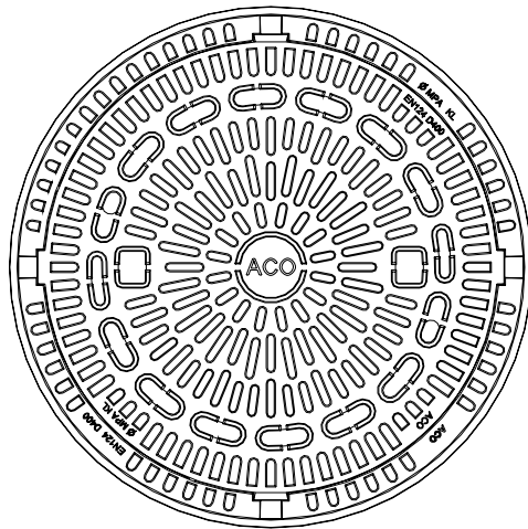
Multitop® Abdeckung mit BEGU® Rahmen rund und Deckel mit Lüftung
