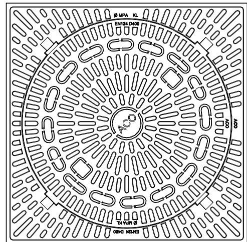
Multitop® Abdeckung mit BEGU® Rahmen eckig und Deckel mit Lüftung
