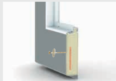
Montage des Lichtschachts ohne Wärmebrücken im Montagekern
