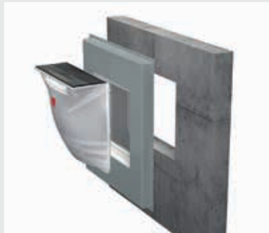
ACO Therm® Block druckwasserdichte Ausfüh- rung mit integriertem hochwasserdichtem ACO Therm® Fenster
