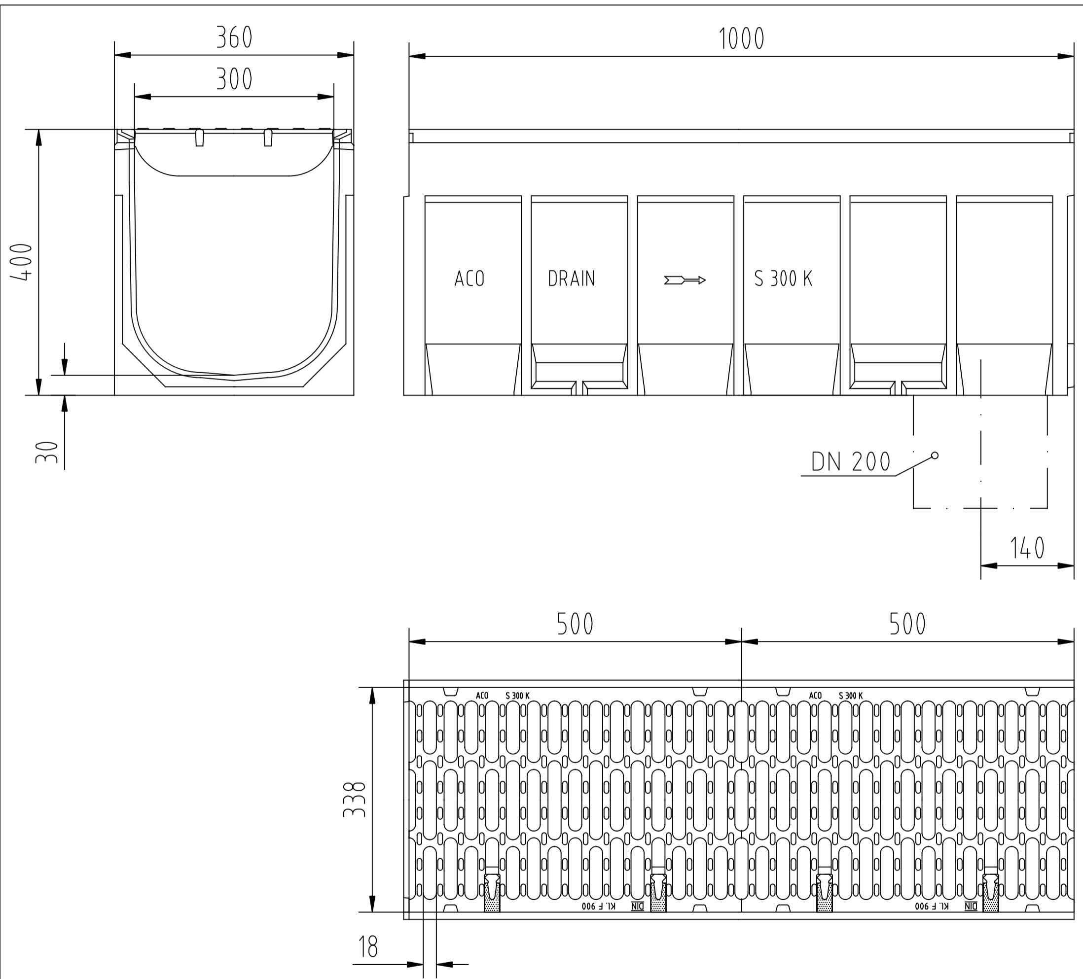
ACO DRAIN Rinne S 300 K mit Gussrost, Art.-Nr. 02700
