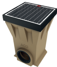
Hofablauf aus Polymerbeton mit Maschenrost (Stahl verzinkt, MW 32x10 mm) und Gusszarge
