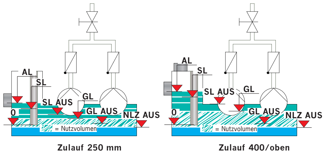
Abb. 5: Schemadarstellung Niveauschaltung
