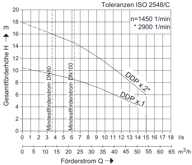
Abb. 7: Kennlinien
