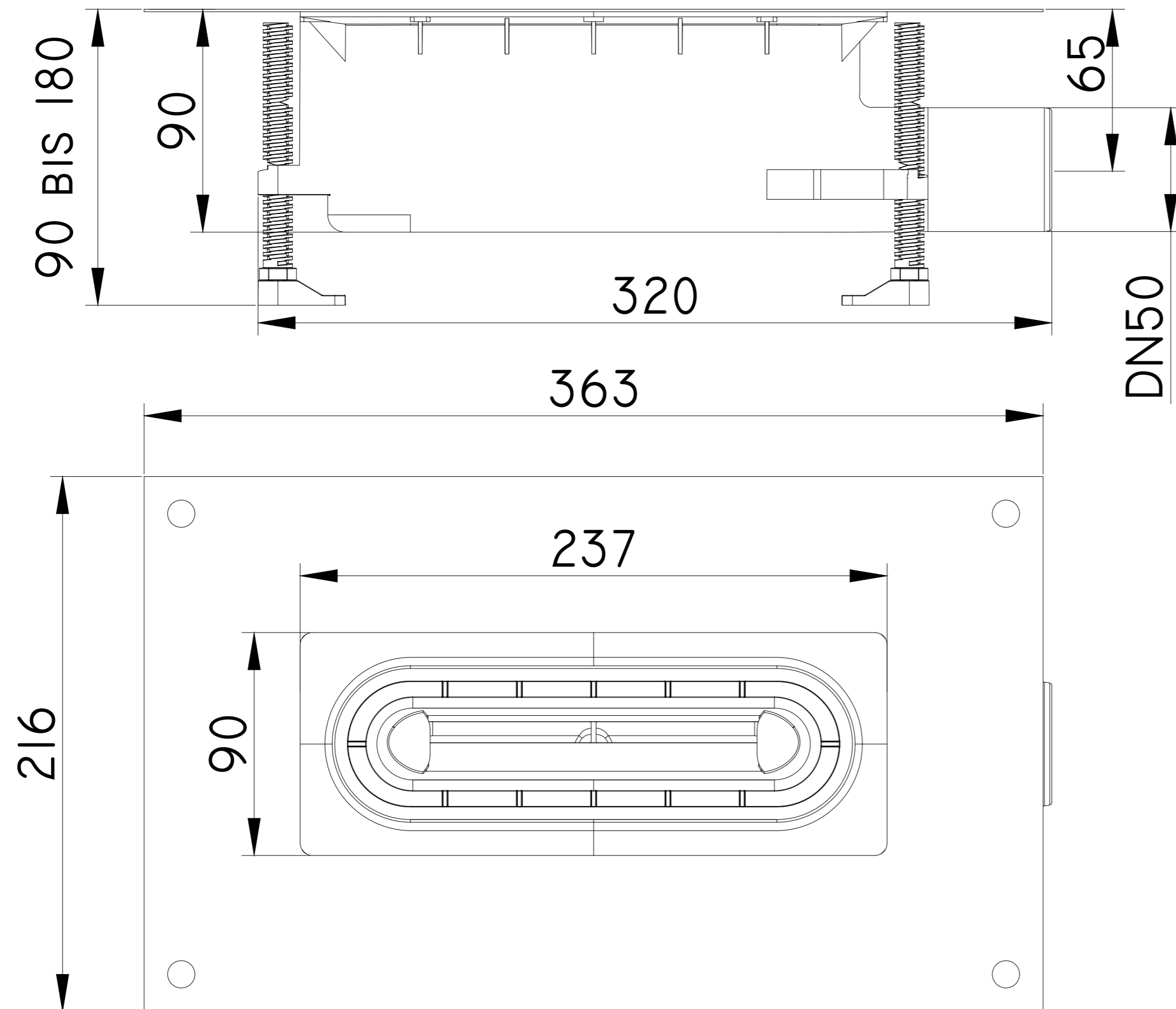
Art.Nr. 9010.51.20 ShowerDrain S+ Rohbauset zu Duschrinnenprofil
